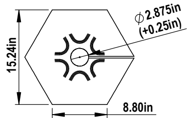
2 16" HELIX N.T.S.
