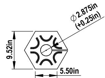
2 10" HELIX N.T.S.
